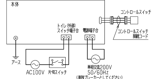
■ 結線図
