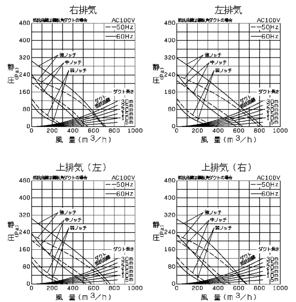
P-Q特性図
