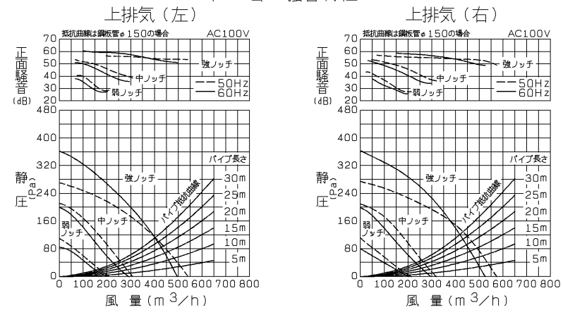
P-Q・騒音特性図
