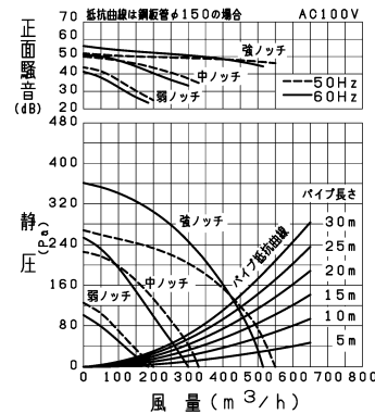
P-Q・騒音特性図
