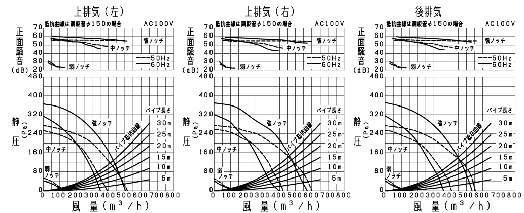
P-Q・騒音特性図
