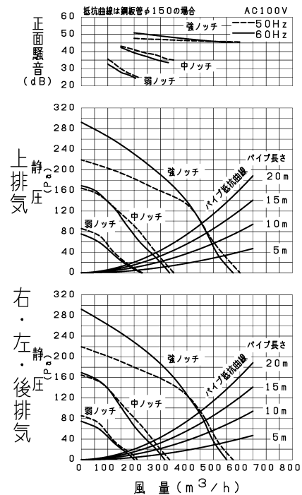
P-Q・騒音特性図
