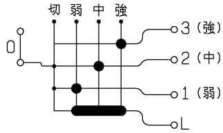
風量切替えスイッチの接点状態
