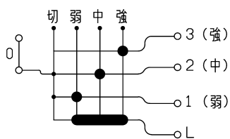
風量切替えスイッチの接点状態
