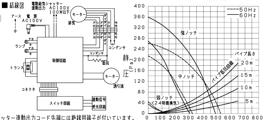
P-Q特性図
