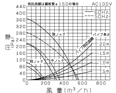
P-Q特性図
