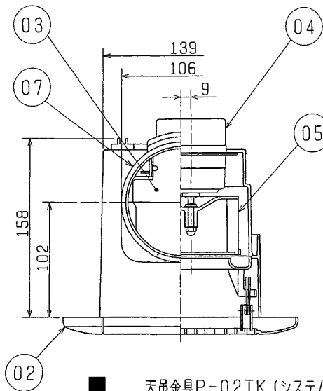
■ 天吊金具P-02TK (システム部材) 取付位置 (2点吊り)
