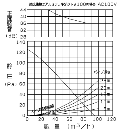
P-Q・騒音特性
