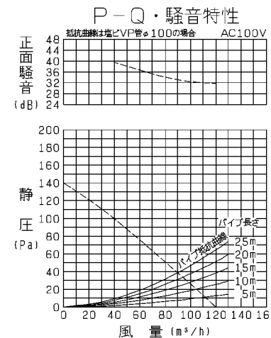
正面騒音は、室外側ダクト内音が測定室に出ないようにし、グリル正面(下方)より1m離れた地点でのAレンジによる値です。
