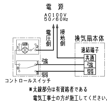
■ 結線図
