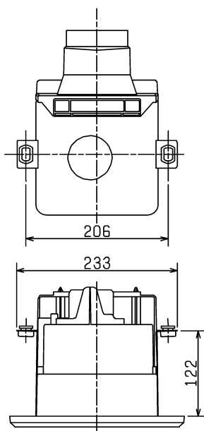
■ 天吊金具P-02TK (別売システム部材) ■ 結線図 据付位置 (2点吊り)
