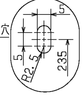
■ 取付穴詳細図
