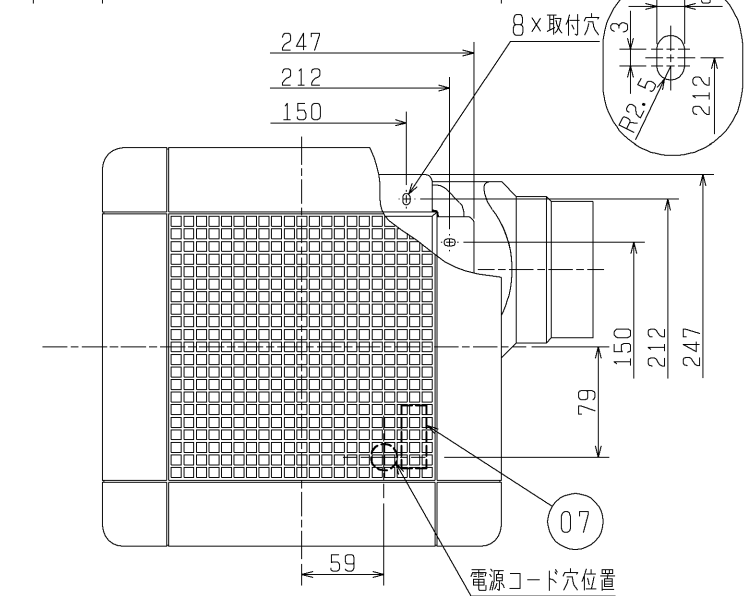
■ 取付穴詳細図
