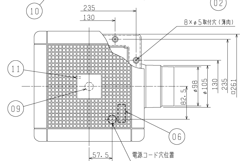
■ 天吊金具P-02TK (システム部材) 取付位置(2点吊り)
