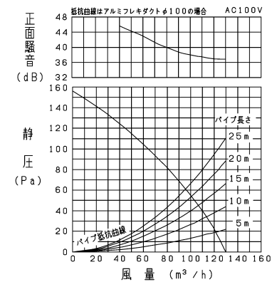
P-Q・騒音特性
