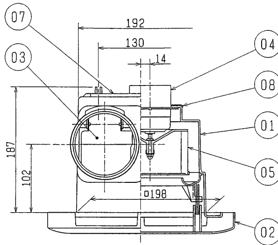
■天吊金具P-Q2TK (システム部材) 取付位置 (2点吊り)
