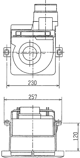
■天吊金具P-Q2TK (システム部材) 取付位置 (2点吊り)
