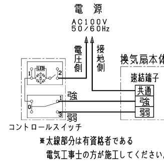
■ 結線図
