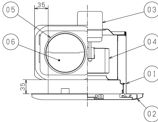
■ 天吊金具P-03TK 2 (別売システム部材) 据付位置 (2点吊り)
