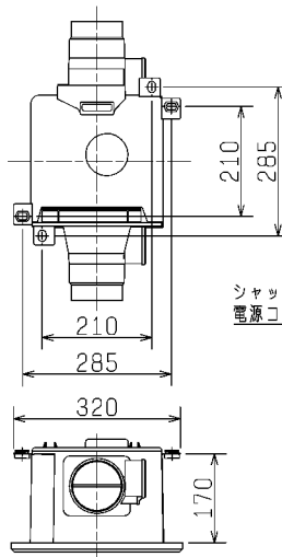
■ 天吊金具P-06TK (別売システム部材) 据付位置(2点吊り)
