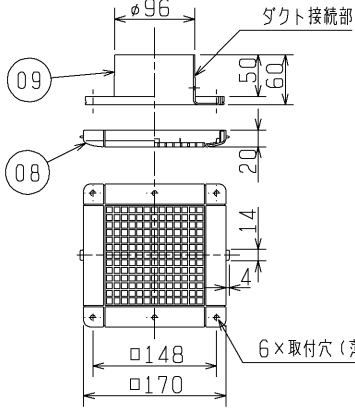
■ 副吸込口グリル (同梱品)
