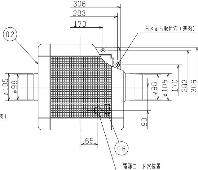
■ 天吊金具P-06TK (システム部材) 取付位置 (2点吊り)
