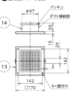
■ 副吸込グリル(同梱)
