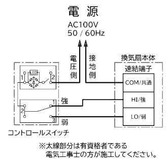
■ 結線図
