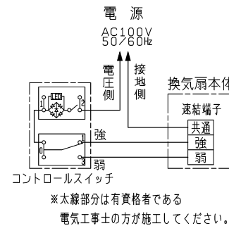
■ 結線図
