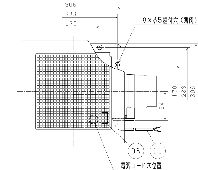
■ 天吊金具P-04TKタイプ (別売システム部材) 据付位置 (2点吊り)
