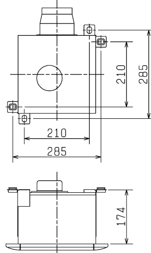
■天吊金具P-05TK (システム部材) 取付位置(2点吊り)
