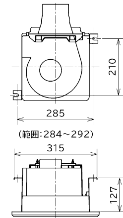
■ 天吊金具P-02TKタイプ (別売システム部材) 据付位置(2点吊り)
