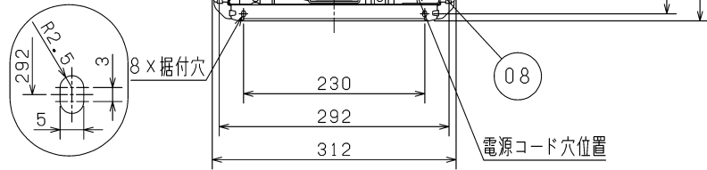
■ 据付穴詳細図
