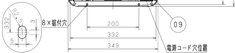
■ 据付穴詳細図
