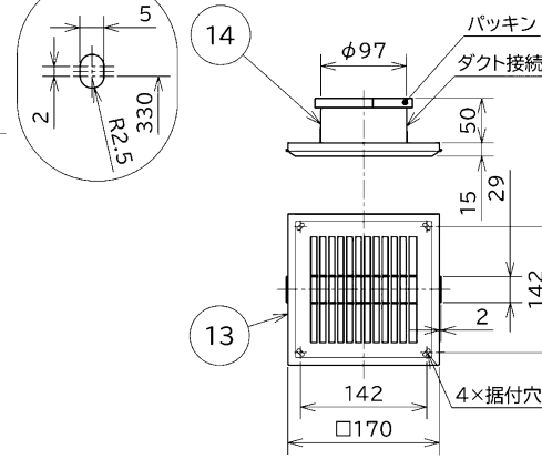
■ 据付穴詳細図 ■ 副吸込グリル(同梱品 2個、出荷時風量割合 開口率100%)
