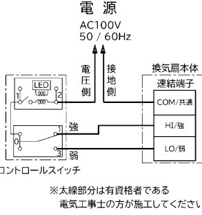
■ 結線図
