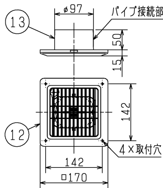
■副吸込グリル(同梱品 2個、出荷時風量調整 開口率100%)
