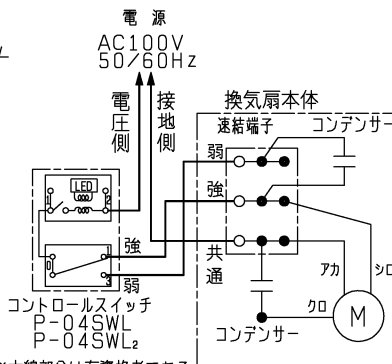
■結線図
