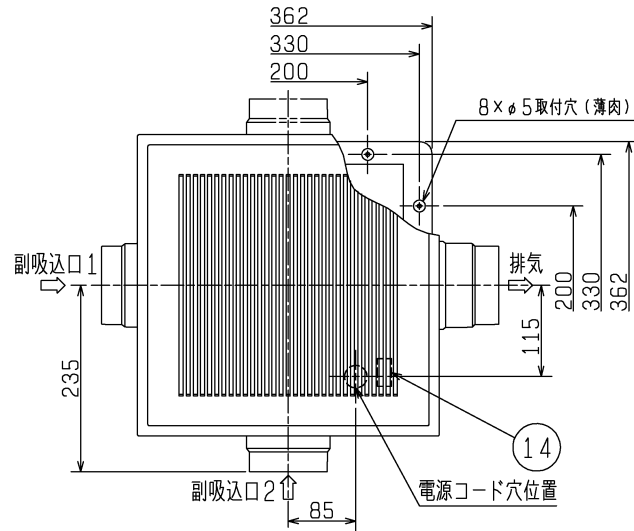
■副吸込グリル(同梱品 2個、出荷時風量調整 開口率100%)
