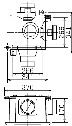
■天吊金具P-06TK(別売システム部材) 取付位置(2点吊り)
