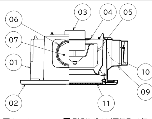
■ 据付穴詳細図
