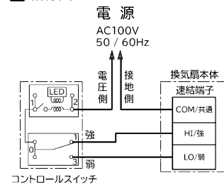
■ 結線図
