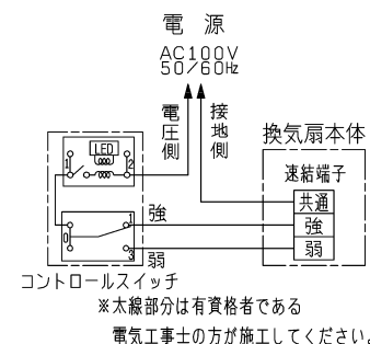
■ 結線図
