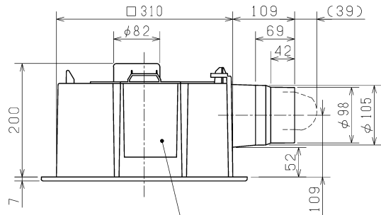
08 本体取付品3個
