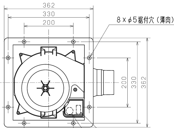
07 電源コード穴位置
