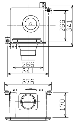
■ 天吊金具P-06TK (システム部材) 取付位置 (2点吊り)
