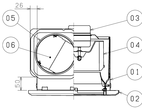
■ 天吊金具P-08TKタイプ ■ 結線図 (別売システム部材) 据付位置(4点吊り)
