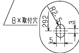
■ 取付穴詳細図
