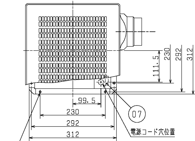
■ 取付穴詳細図
