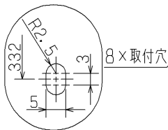
■ 取付穴詳細図
