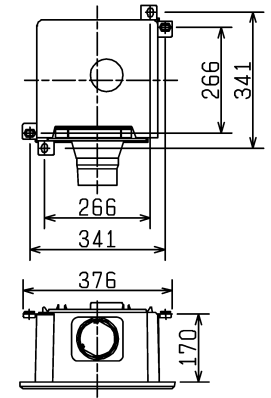
■ 天吊金具P-06TK (別売システム部材) 据付位置(2点吊り)
