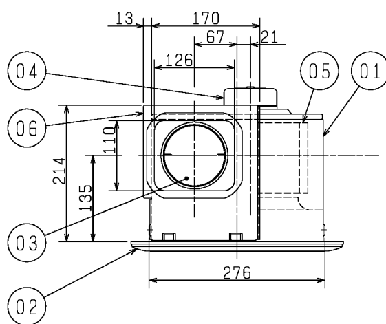
■ 天吊金具P-08TK (システム部材) 取付要領図 (4点吊り)
