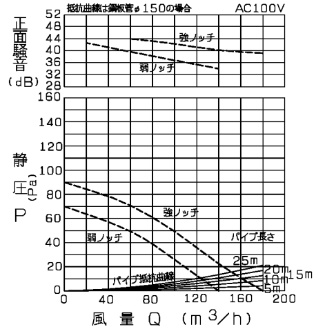
P-Q・騒音特性(排気時)
