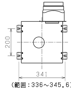
■ 天吊金具P-08TKタイプ (別売システム部材) 据付位置(4点吊り)
