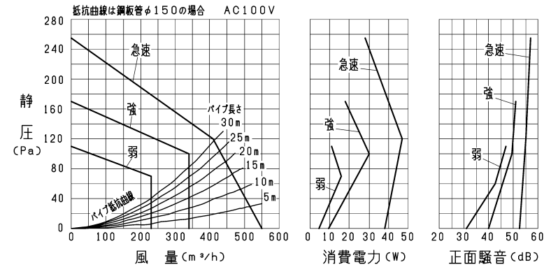
P-Q・消費電力・騒音特性
