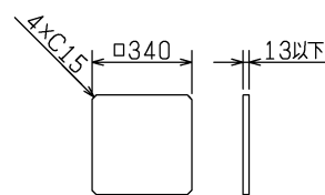
■ 天井材寸法
