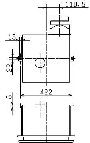
■ パネル寸法
