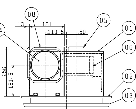
■ 取付図
