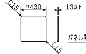
■ パネル寸法
