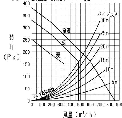
抵抗曲線は鋼板管φ150の場合 AC100V
