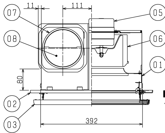
■ 天井金具P-08TK (システム部材) 据付位置 (4点吊り)
