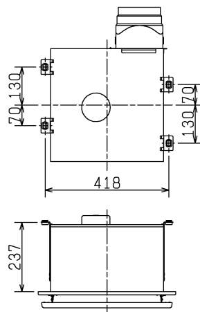
■ 天井金具P-08TK (システム部材) 据付位置 (4点吊り)
