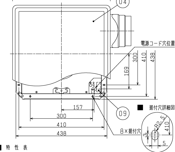
■ 天井金具P-08TK (システム部材) 据付位置 (4点吊り)
